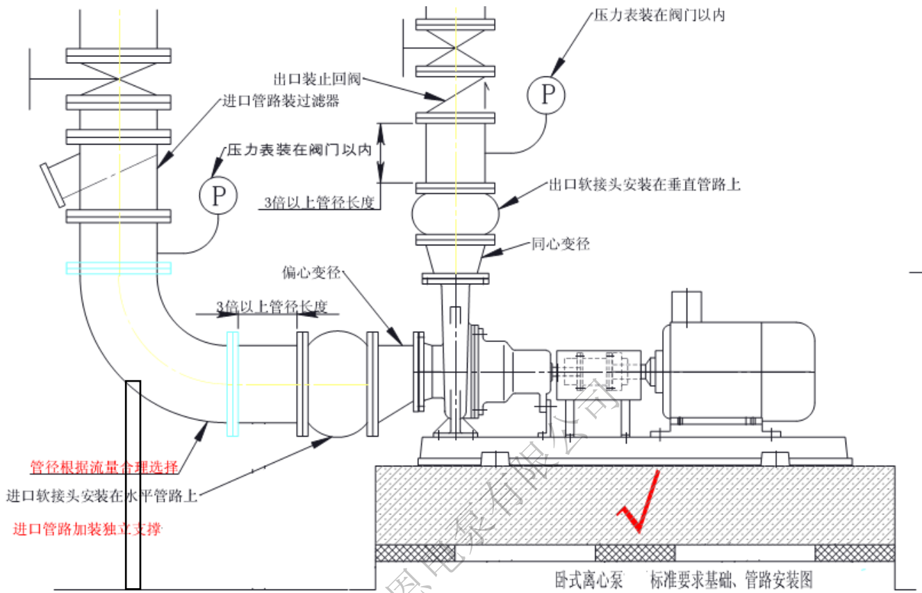
泵管路安装要点示意图
